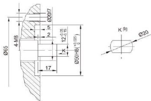
轴伸结构 BB-B25A-1
